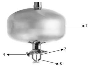
Sistema modular
